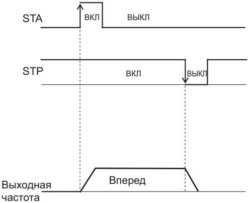
(2) Используются STA и STP
