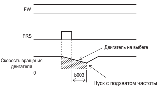
(Пример 2) Перезапуск с подхватом частоты
