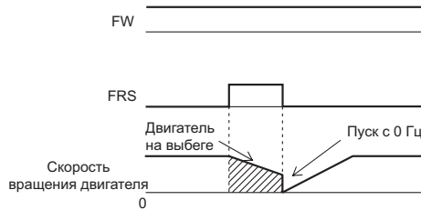
(Пример 1) Перезапуск с 0 Гц
