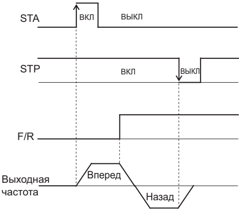
(1) Используются STA, STP и F/R
