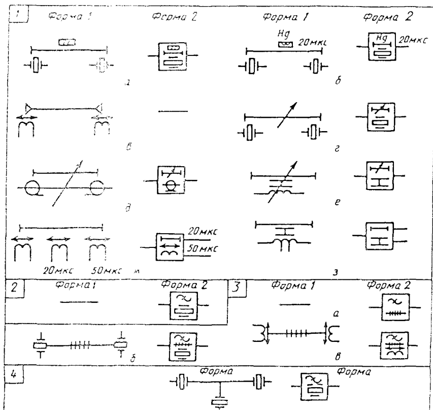
2.17. Устройства связи (ГОСТ 2.737–68)
