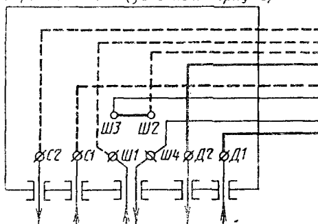
Коробка выводов (условно повернута)
