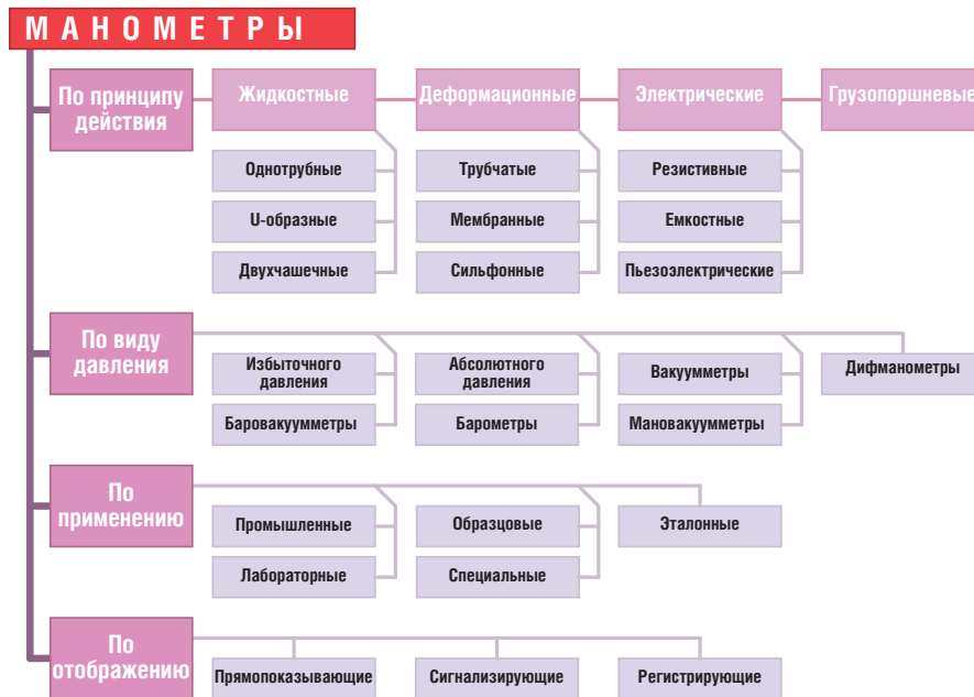
Рис. 3. Классификация манометров
