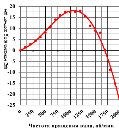
Рис. 6. Экспериментальная характеристика N=f(n) модели микроГЭС
