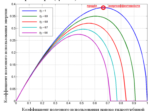
Рис. 2. Графическая иллюстрация предела энергетической эффективности
