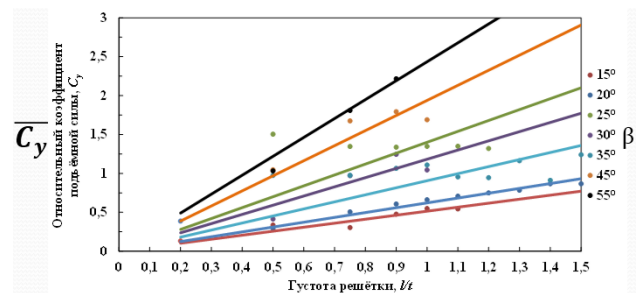
Рис. 4. Номограмма C_y=f(l/t, \beta) , полученная расчётно-экспериментальным методом
