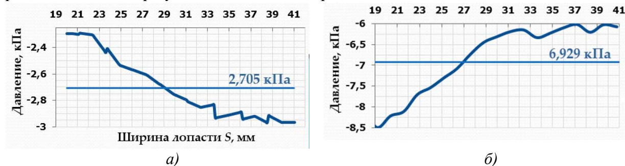
Рис. 10. Эпюры распределения давления в межлопастном канале рабочего колеса. а - на входе, б - на выходе
